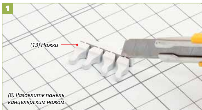
1 При помощи канцелярского ножа отделите ножки (13) и панели (8), обработайте их края наждачной бумагой.
