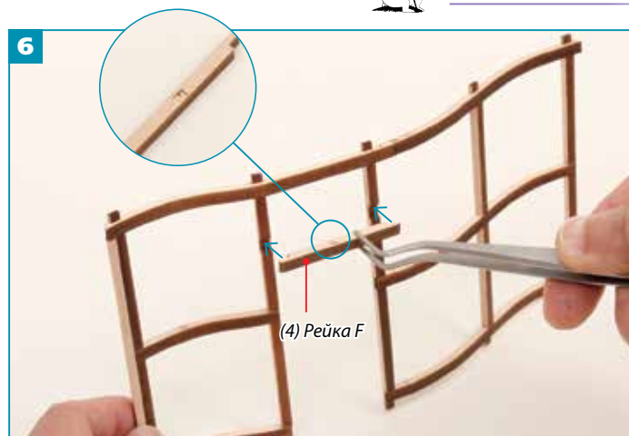
6 При помощи клея для дерева прикрепите рейку F, как показано выше.
